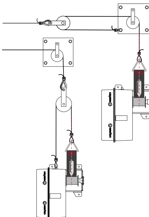
Fig. 06.13. Ejemplo. Instalación de GOLIAT con cincha y polipasto.
