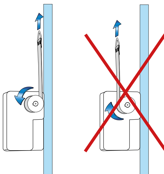
Fig. 06.12. Posición y dirección de la cincha.
