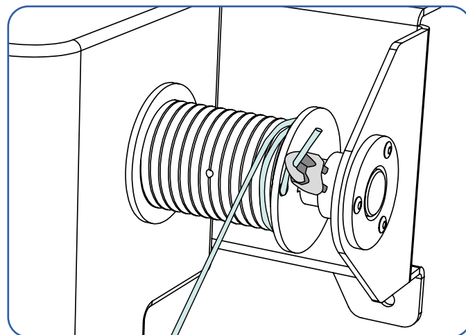
Fig. 06.01-B. Anclaje de la sirga al carrete.
