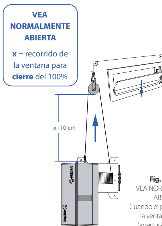
Fig. 06.07. VEA NORMALMENTE CERRADA. Cuando el polipasto sube la ventana se cierra (apertura del 0%).
